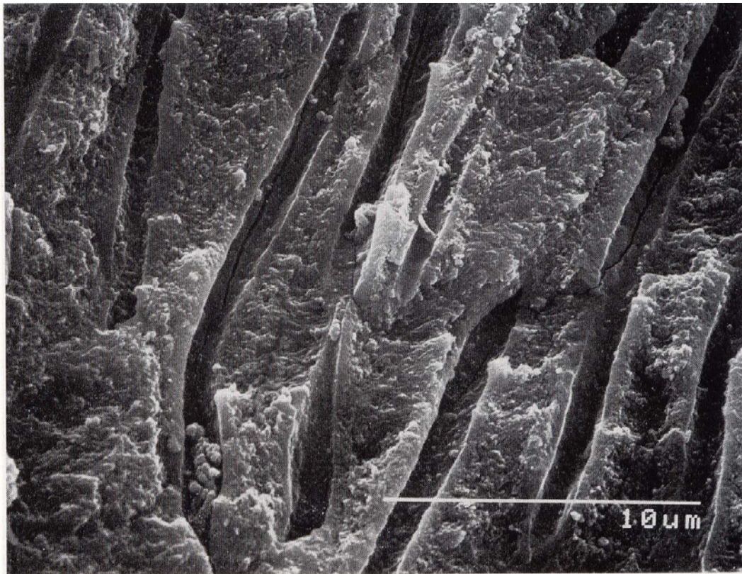
図 25 フッ素イオン導入群;露出象牙質最表層から約 300 \mu\text{m} 深層の象牙質断面 SEM 像 (弱拡大)
