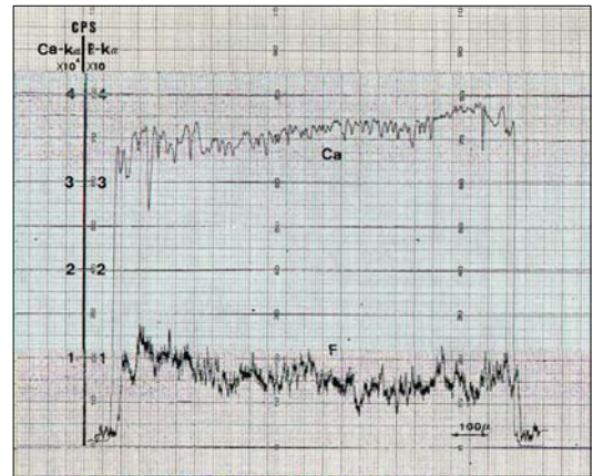
図4 対照群におけるF、Ca元素の線分析 (線分析はすべて右側が露出象牙質最表層である)
